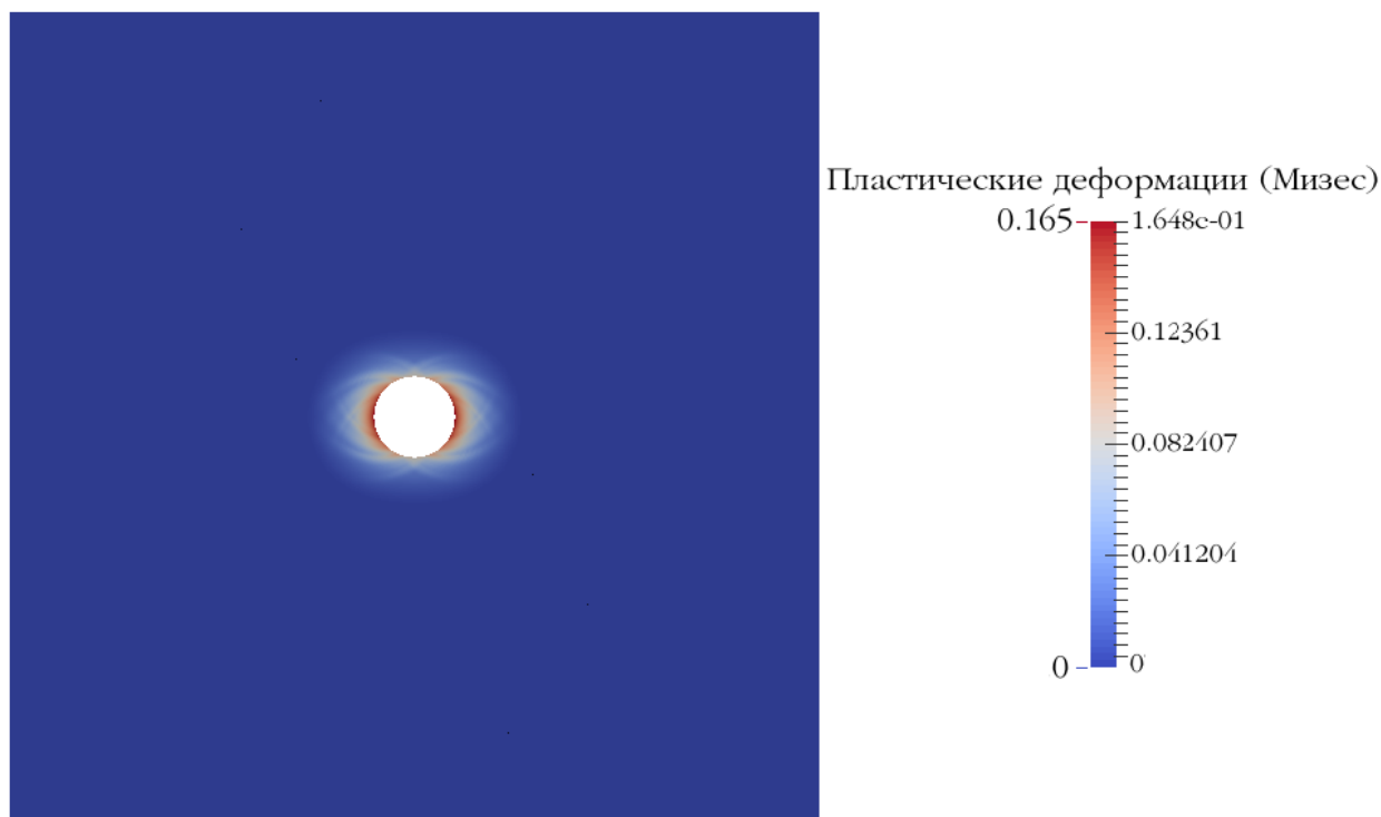
Результаты- Пластические деформации на полной пластине (другая цветовая схема)
