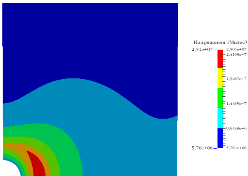
Результаты - Напряжение Мизес
