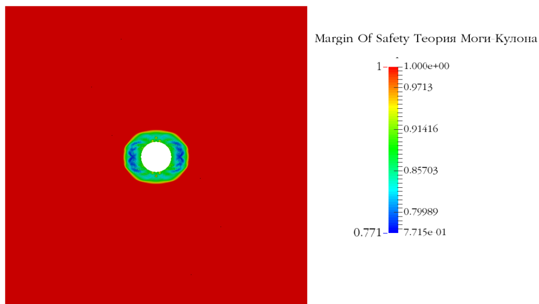
Результат расчета запаса прочности по теории Могги-Кулона
