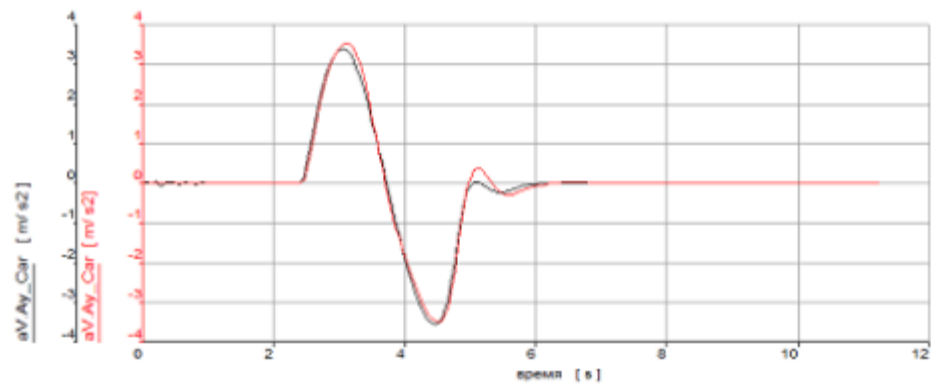
Рис. 12: Боковое ускорение для жесткой и упругой рамы на скорости испытания 55 км/ч.
