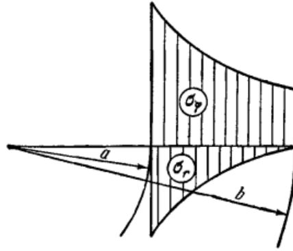
Рисунок 1. Распределение напряжений по толщине стенки
